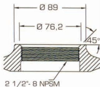
Priključak za tank 2 1/2"
