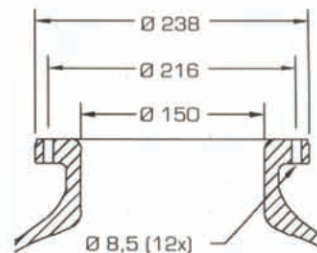
Priključak za tank 6"
