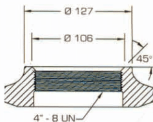
Priključak za tank 4"
